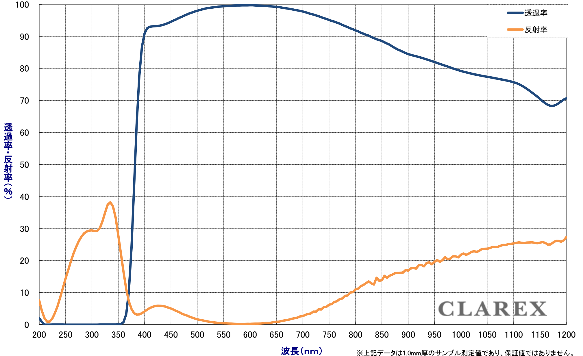
ARフィルター 両面ARコート (片面撥水コート) 分光透過率・反射率(%)
